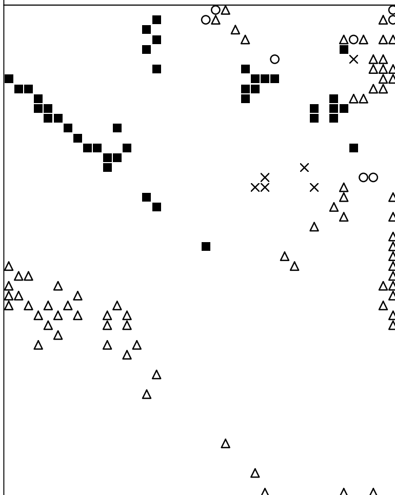
Basisplaat 6 410 = ■ 411 = ○ 412 = × 414 = △
