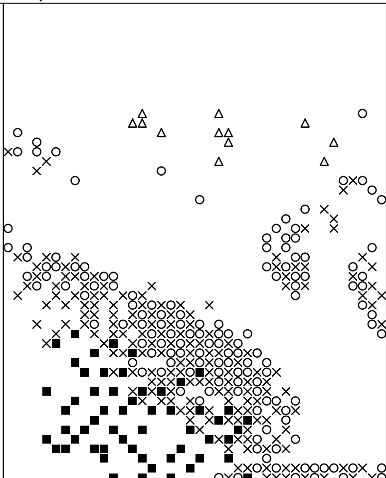
Basisplaat 6 376 = ■ 388 = ○ 407 = × 409 = △
