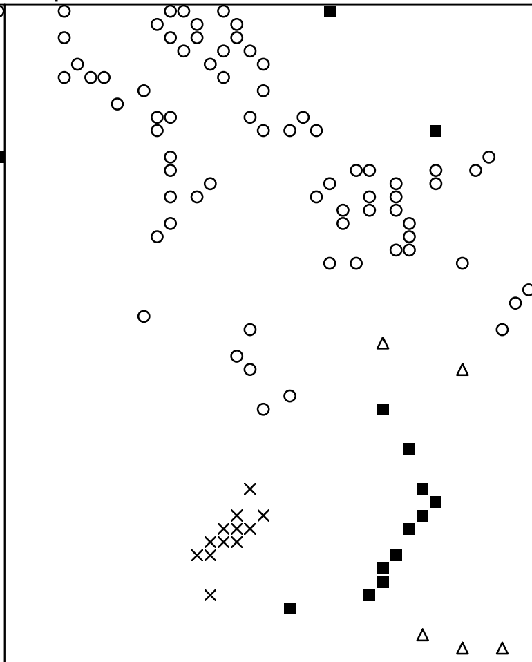
Basisplaat 11 143 = ■ 164 = ○ 167 = × 172 = △
