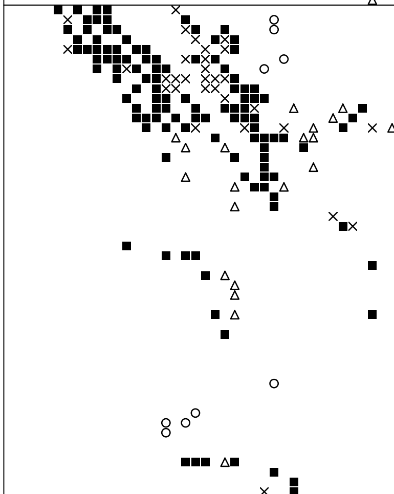
Basisplaat 11 173 = ■ 175 = ○ 185 = × 191 = △
