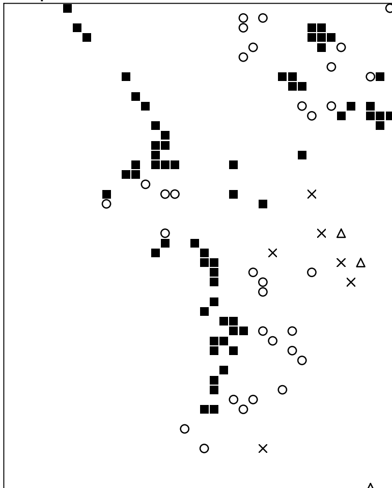
Basisplaat 11 101 = ■ 108 = ○ 115 = × 141 = △
