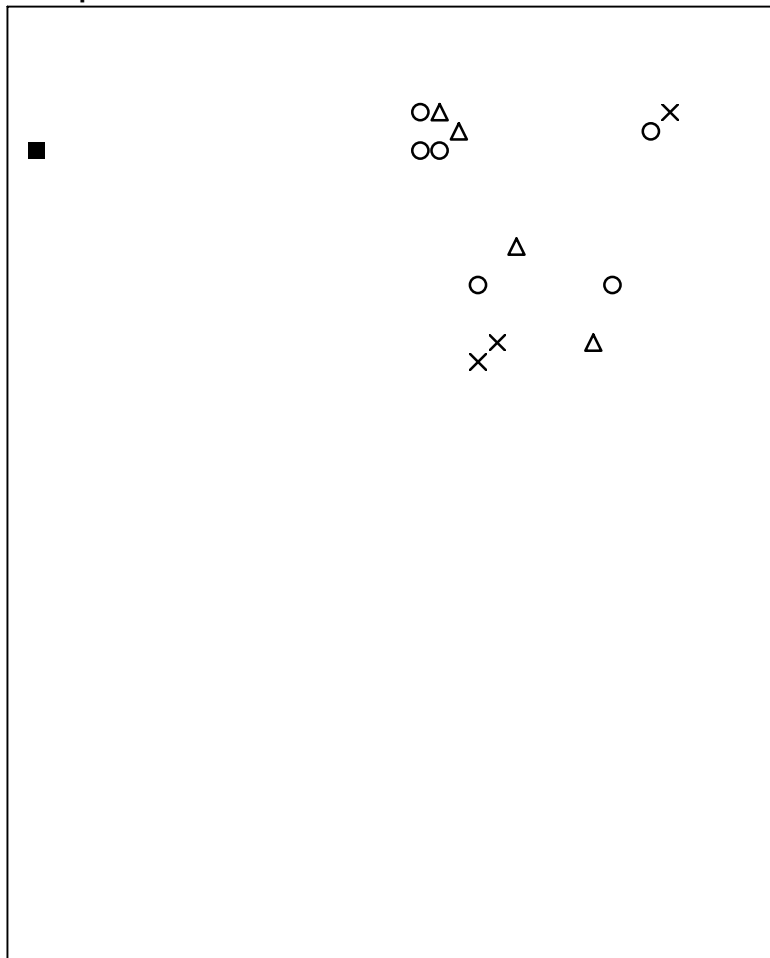
Basisplaat 6 363 = ■ 364 = ○ 365 = × 366 = △
