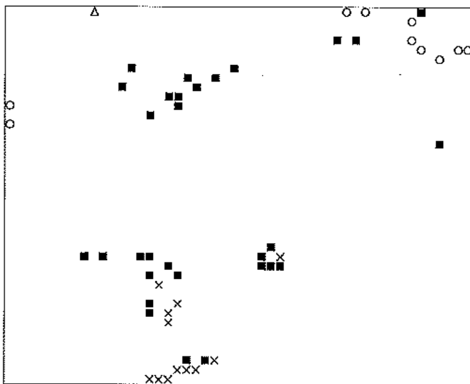
Plaque 4 Couleur de pixel 161 = ■ Couleur de pixel 170 = ○ Couleur de pixel 224 = × Couleur de pixel 227 = △
